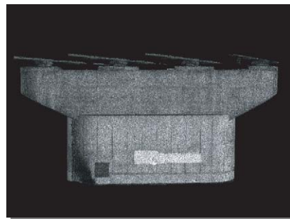
スキャナーデータ (点群)
